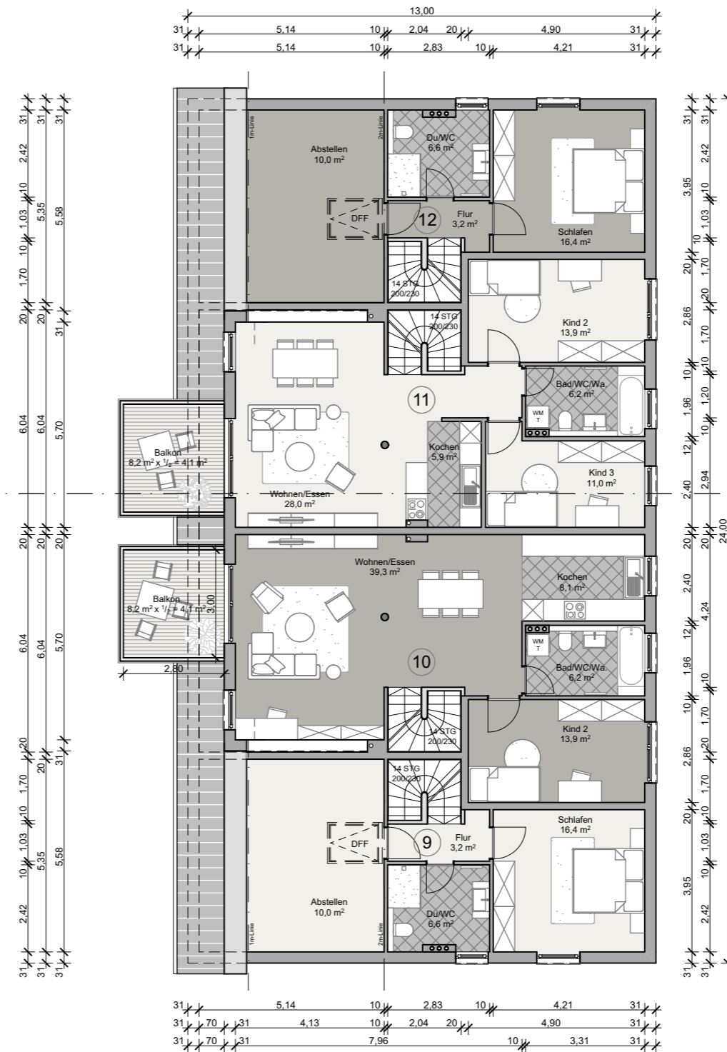
DACHGESCHOSS
