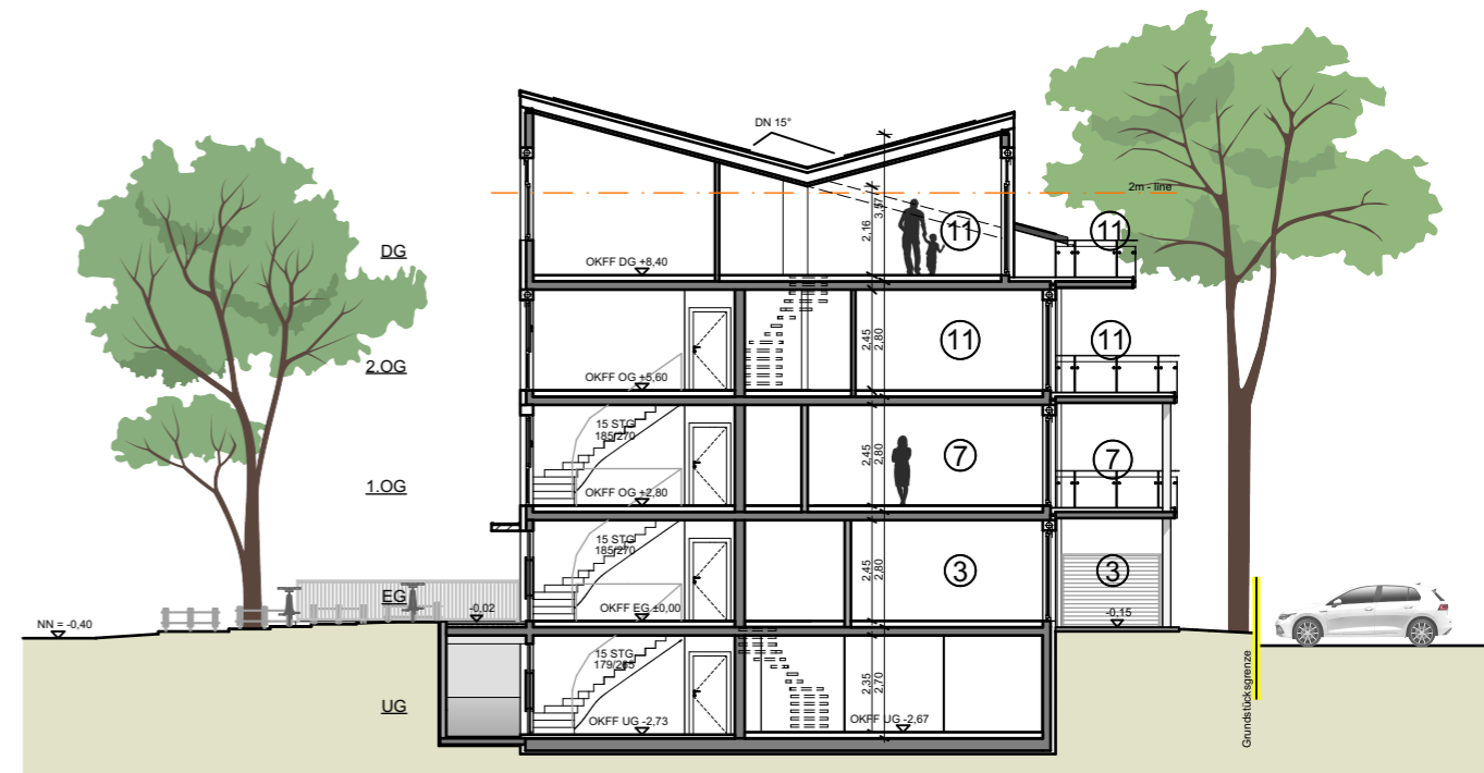
Schnitt A-A
