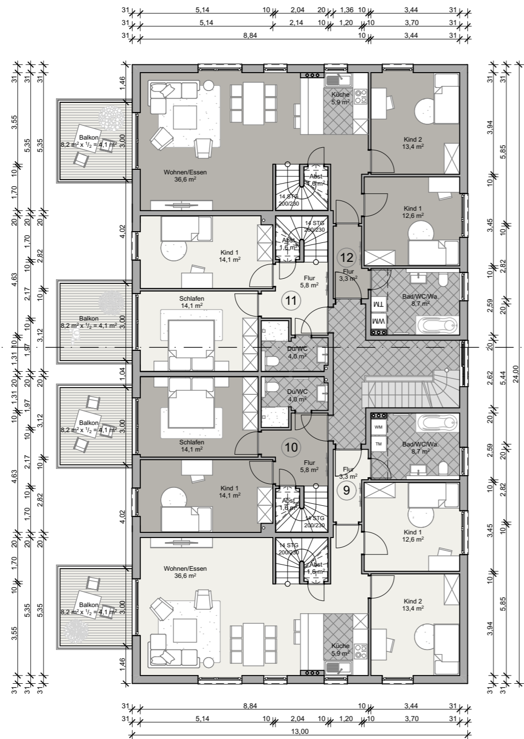
2. OBERGESCHOSS
