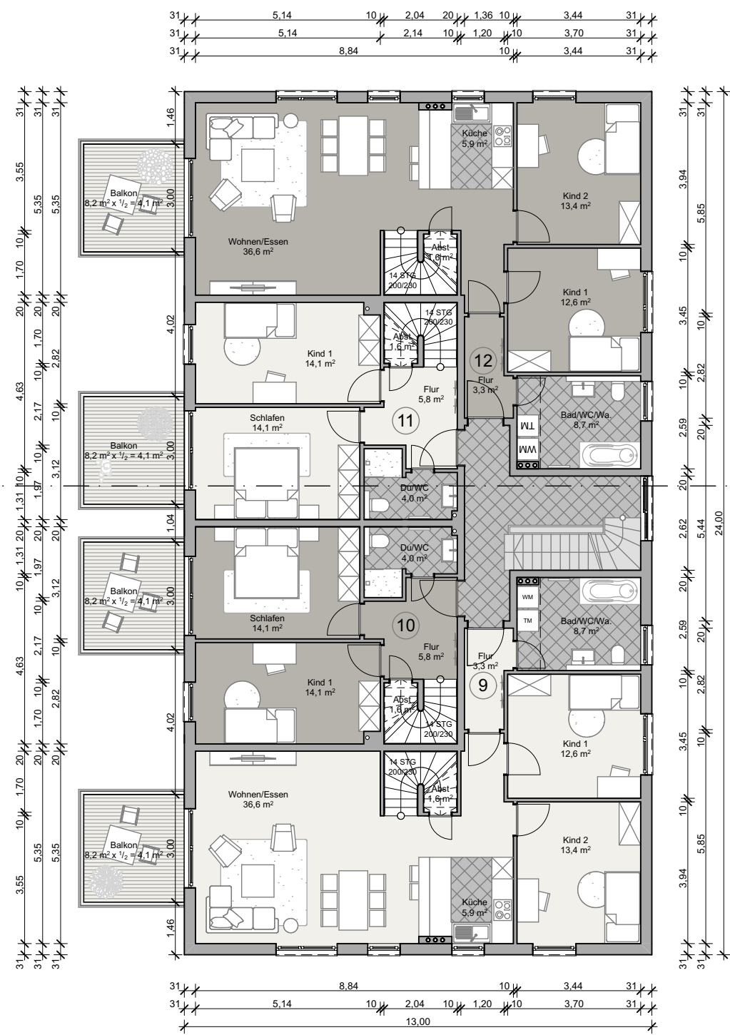
2. OBERGESCHOSS
