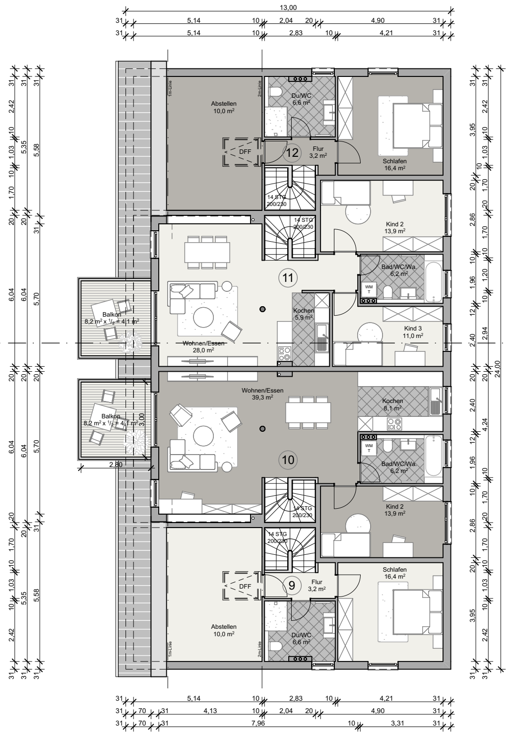
DACHGESCHOSS
