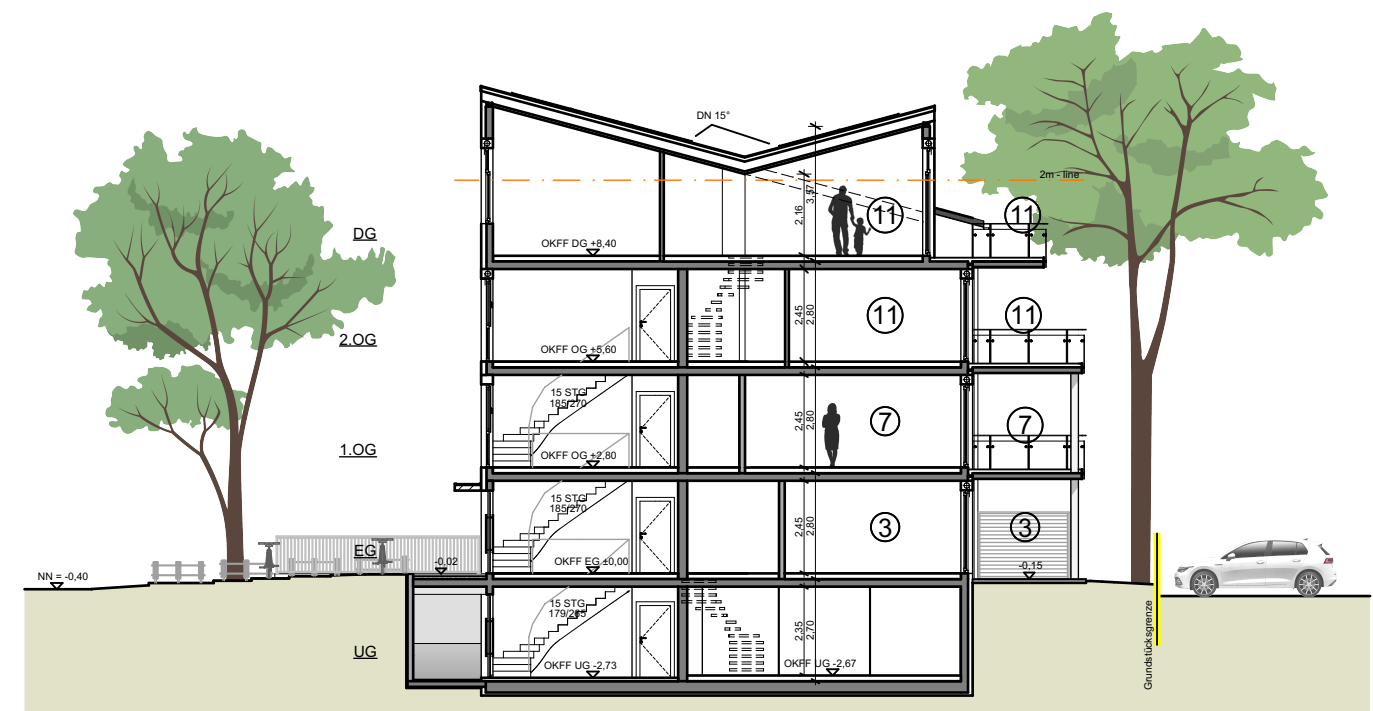
Schnitt A-A
