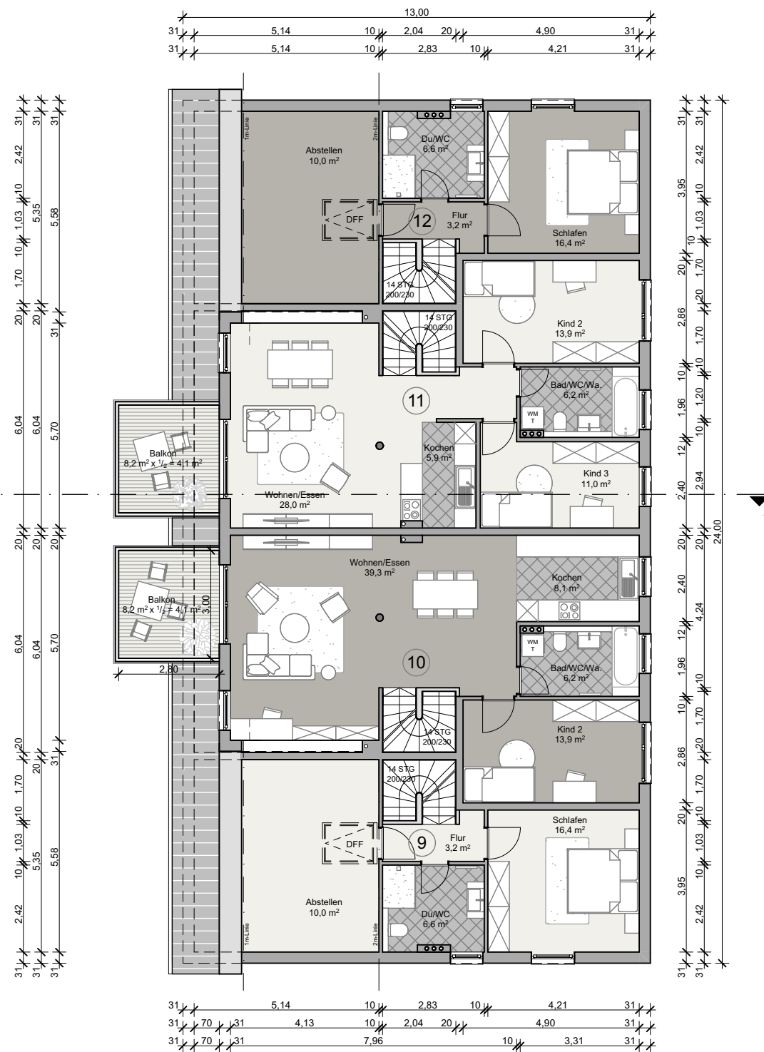
DACHGESCHOSS
